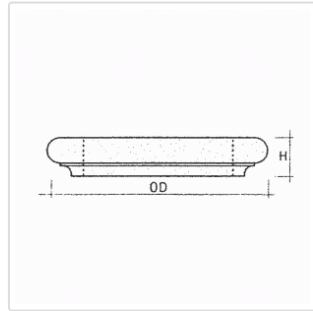
Astragal - CAFA
