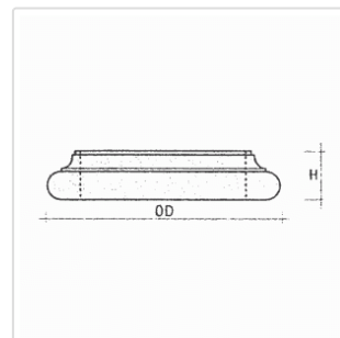
Ornate - CAFO
